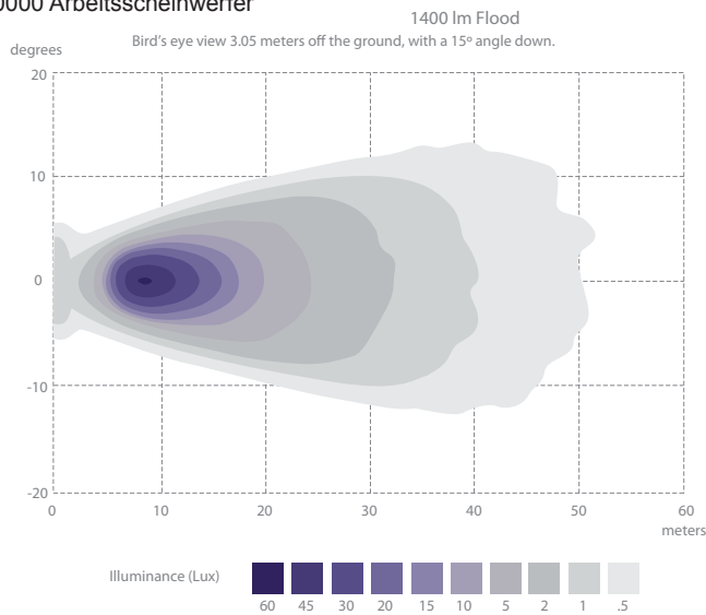
W1500000 Arbeitscheinwerfer
